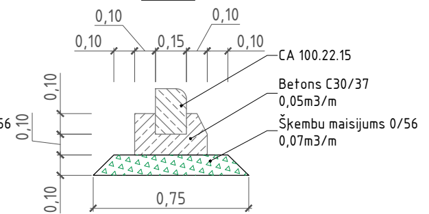
CA 100.22.15 M 1:25
