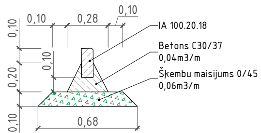
IA 100.20.8 M 1:25
